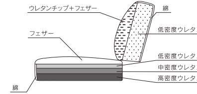
座内部構造図 [3層ウレタン構造]
