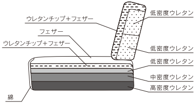
座内部構造図 [3層ウレタン構造]
